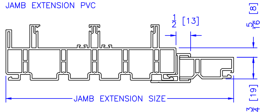
JAMB EXTENSION PVC
