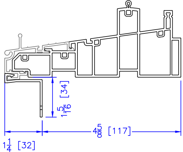
NAILING FIN
