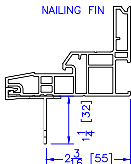
NAILING FIN
