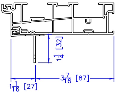
NAILING FIN
