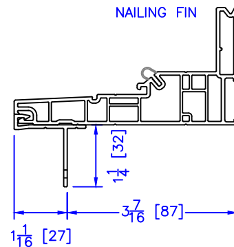
NAILING FIN
