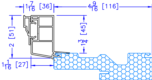
2" RENO DOOR BM
