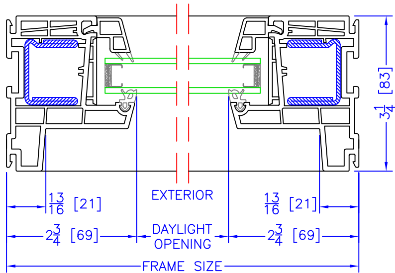
JAMBS
