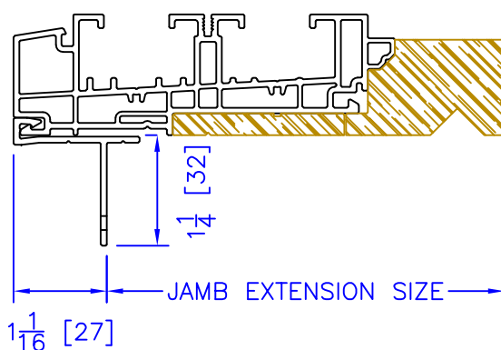
NAILING FIN
