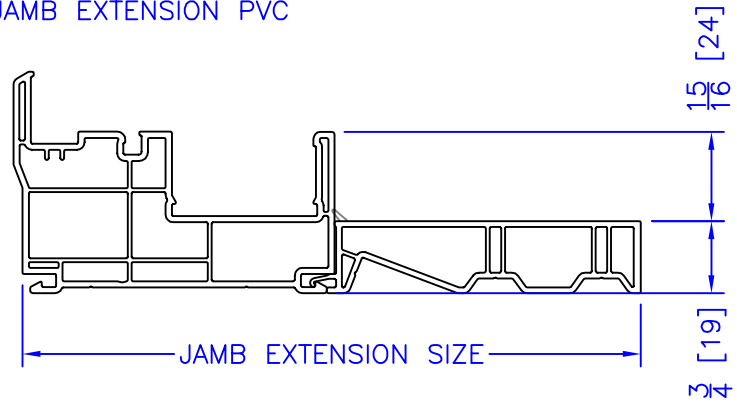
JAMB EXTENSION PVC
