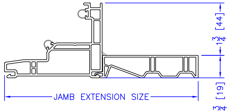
JAMB EXTENSION PVC
